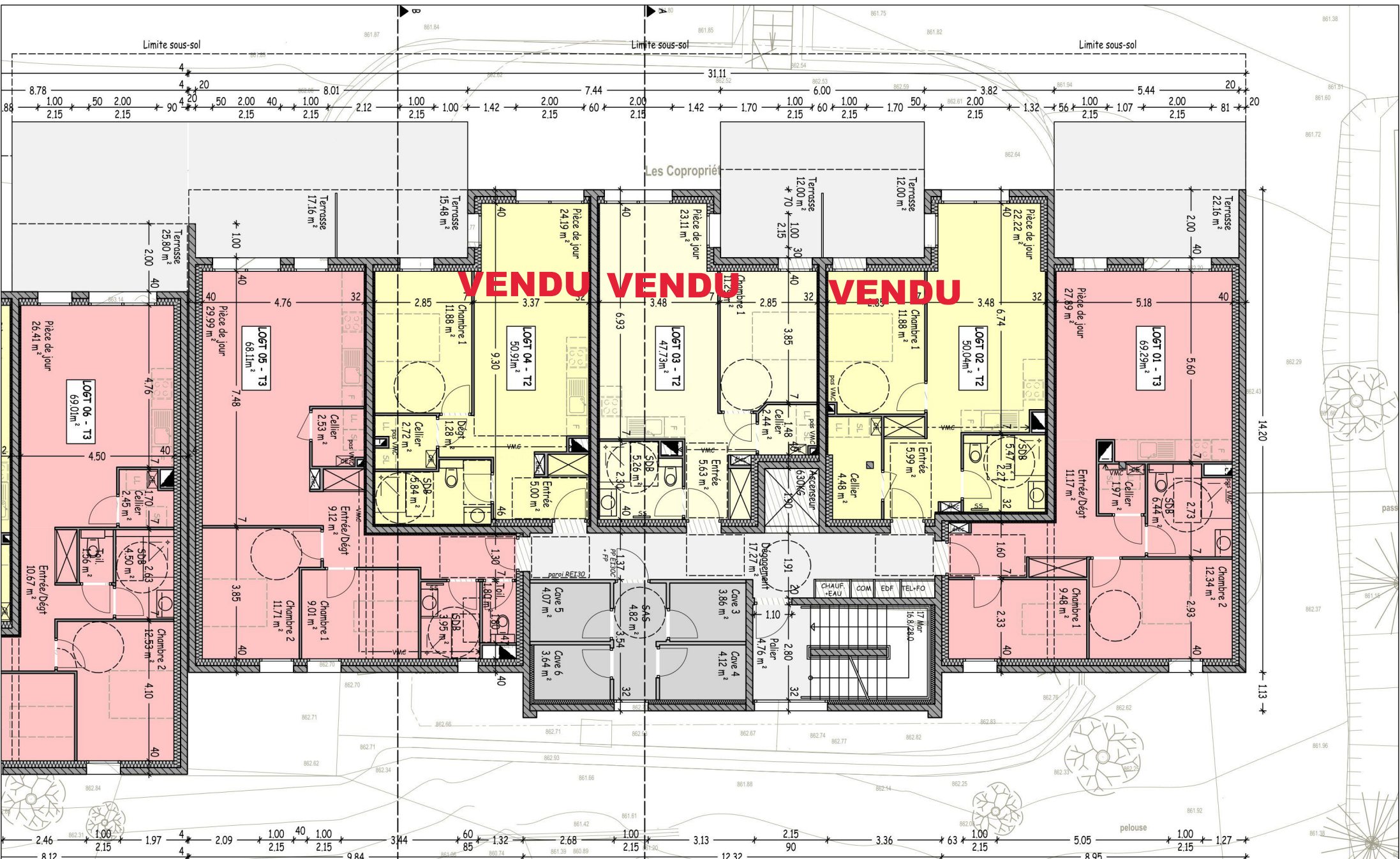
NIVEAU RDJ BATIMENT A - 1/100e
